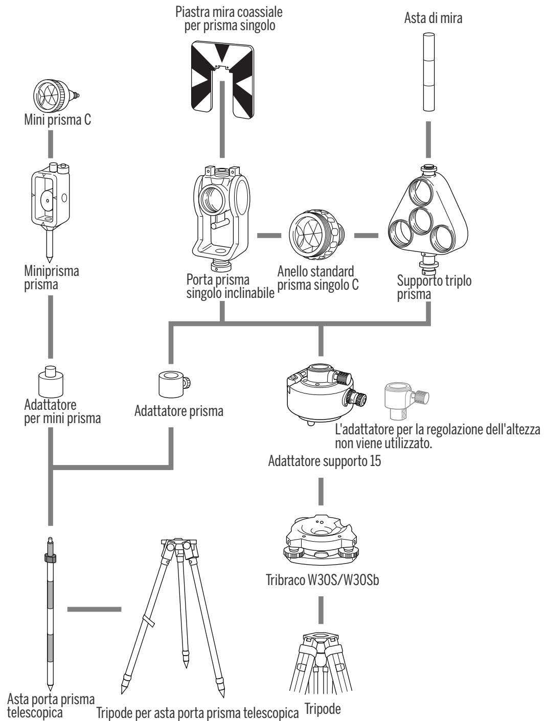
Figura 5.2 Prisma, lato riflettente
